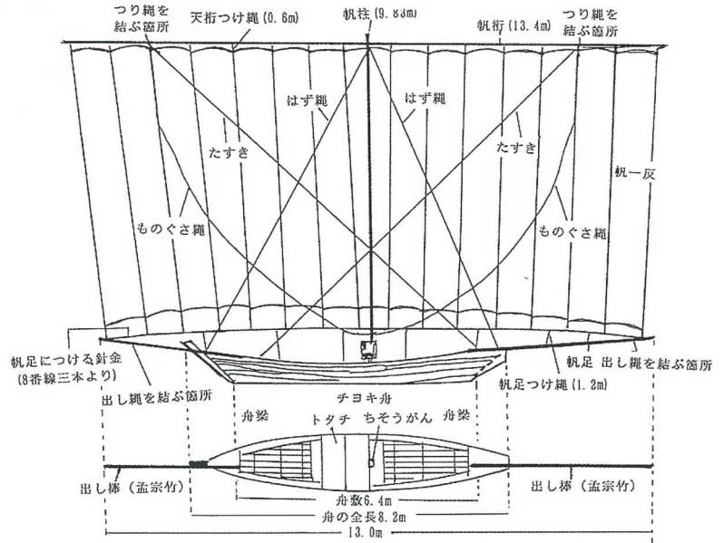
▲霞ヶ浦の帆曳舟概要図
