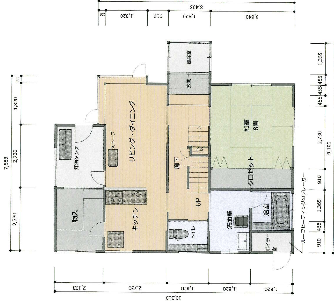
1階縮尺 1/100
