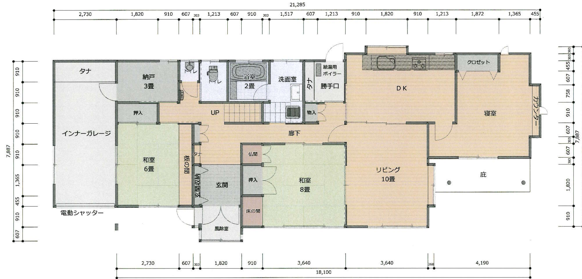
1階縮尺 1/100
